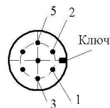
Рисунок 5 Схема расположения контактов
