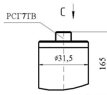
Рисунок 3 С разъемом Остальное см. рисунок 1,4
