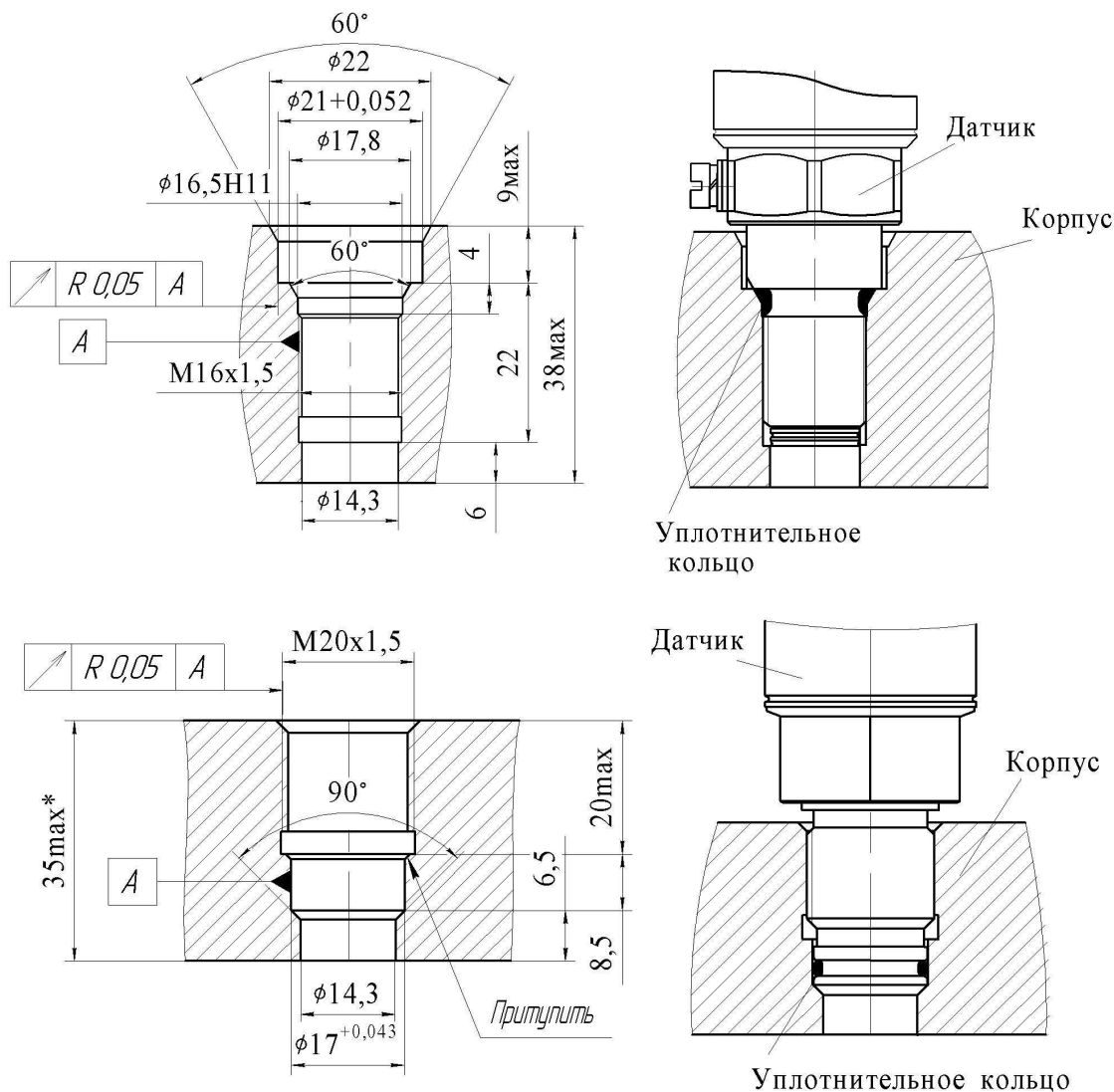
Рисунок 6 –Разметка монтажного гнезда и установка датчика МИДА-ДИ-12П-072-К
