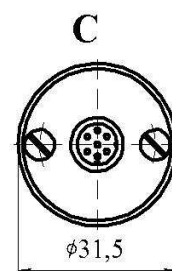
Рисунок 5 Схема расположения контактов
