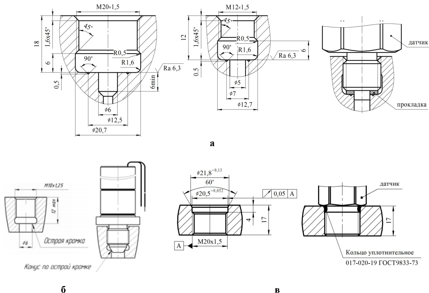
Рисунок 4 - Разметка монтажных гнезд под датчики и установка датчика на рабочей магистрали: а - для датчиков с приемной полостью (М20, М12); б - для датчиков с уплотнением «конус по острой кромке»; в - для датчиков с открытой мембраной (ОМ20)
