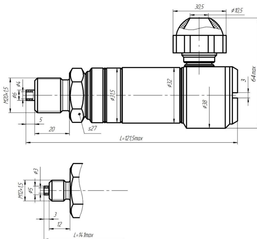
Рисунок Д.10– Габаритные и присоединительные размеры датчиков МИДА-ДИ (ДА, ДВ, ДИВ)-15-УМ, МИДА-ДИ (ДА, ДВ, ДИВ)-15-Ех-УМ с токовым выходным сигналом (код сигнала 01) ), с выходным сигналом в виде напряжения постоянного тока (код сигнала (051, 052, 053, 054, 055, 056, 057) и цифровым выходным сигналом (код сигнала 061-064).
