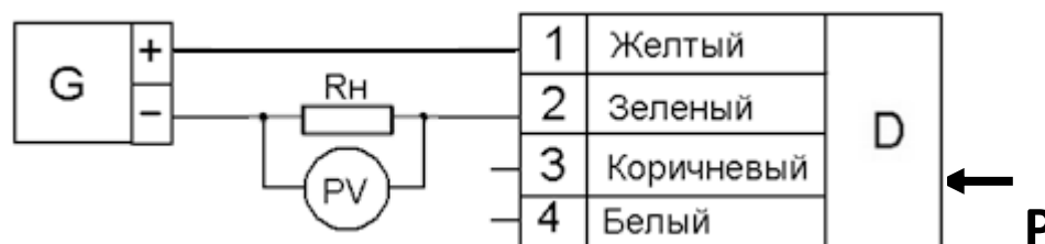
Рисунок Г.5 - Схема включения при проверке и настройке датчиков МИДА-15-А с выходным сигналом в виде напряжения постоянного тока 0,5-4,5 В (код линии 057).
