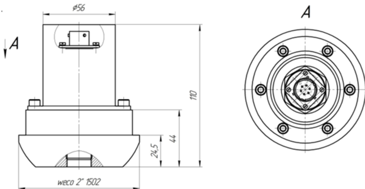
Рисунок Д.19 – Габаритные и присоединительные размеры переходника МИДА-ОМ20х1,5/HU-15021502 (соединение Hammer Union, предназначено для тяжелых условий эксплуатации) с установленным в нем датчиком МИДА-ДИ-15-ОМ20-ПР6.
