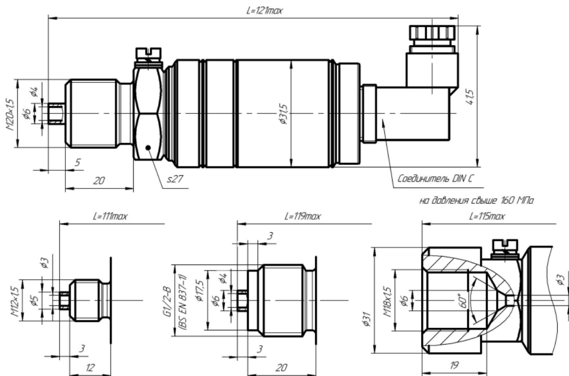
Рисунок Д.1 – Габаритные и присоединительные размеры датчиков МИДА-ДИ (ДА, ДВ, ДИВ)-15, МИДА-ДИ (ДА, ДВ, ДИВ)-15-Ех, МИДА-ДИ-15-М с выходным сигналом в виде напряжения постоянного тока с наличием подстройки «нуля» и «диапазона» (код сигнала 051, 052, 058, 059)
