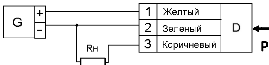
Рисунок Г.4 - Схема подключения датчиков с выходным сигналом в виде постоянного тока 4-20 мА (код линии 01) при проверке и настройке.
