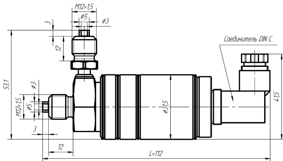
Рисунок Д.2 – Габаритные размеры датчика МИДА-ДД-15, МИДА-ДД-15-Ех с выходным сигналом в виде напряжения постоянного тока и наличием подстройки «нуля» и «диапазона» (код сигнала 051, 052, 058, 059)
