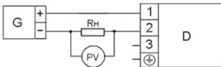
Рисунок В.3 Схема внешних электрических соединений для датчиков с протоколом обмена Mida/UART (код линии 061, 062) в режиме непрерывной периодической передачи информации об измеренном давлении.
