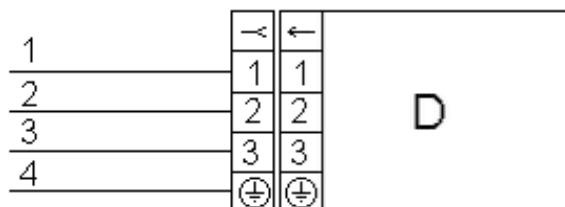
Рисунок В.1 Схема внешних электрических соединений для датчиков с выходным сигналом в виде напряжения постоянного тока (код линии 051, 052, 053, 054, 055, 056, 057, 58, 59)
